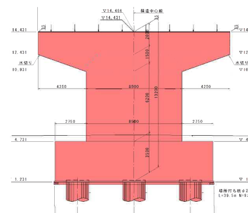
【正面図】
