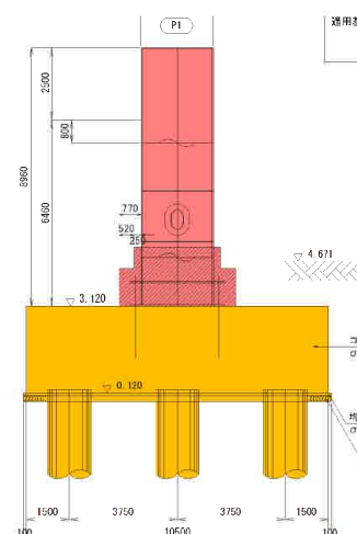
【側面図】(P1)
