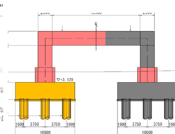
【正面図】(P1)
