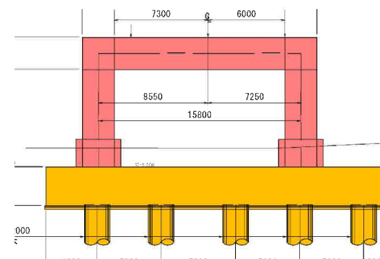
【正面図】
