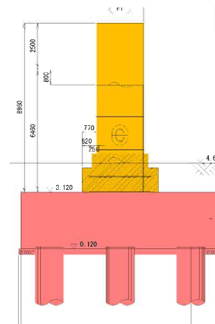
【側面図】(P1)
