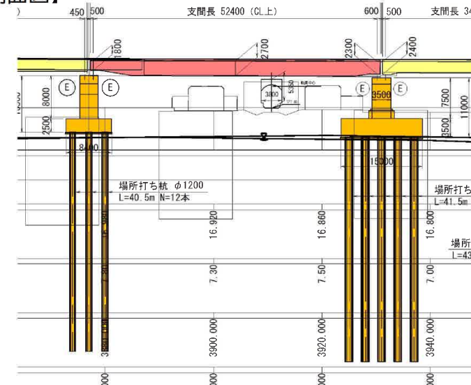
【側面図】
