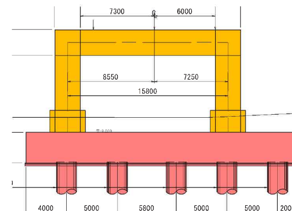
【正面図】(P1)
