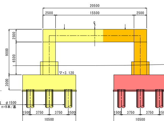
【正面図】
