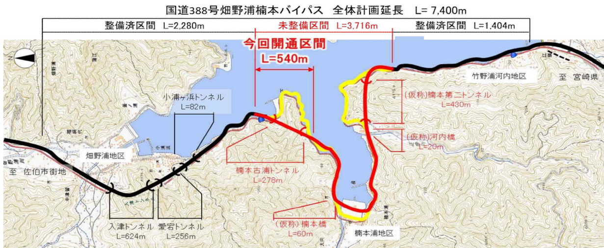
▲平面図
