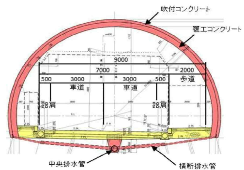
▲トンネル部標準断面図
