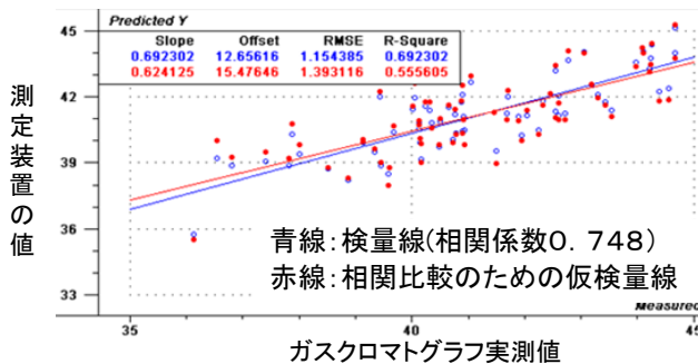
図1 豚専用検量線
