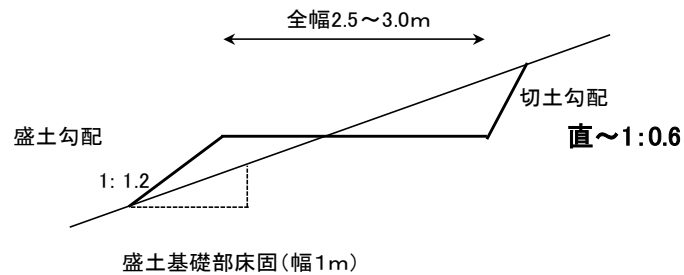
土工標準図
