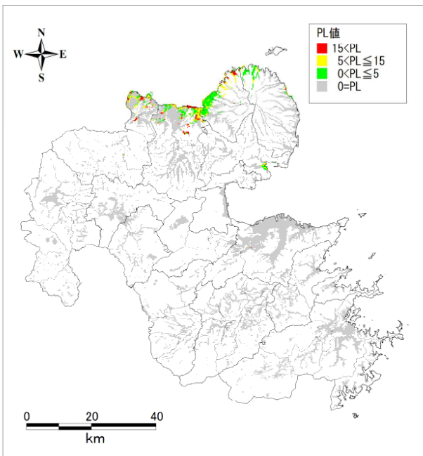
周防灘断層群主部の地震による液状化危険度分布
