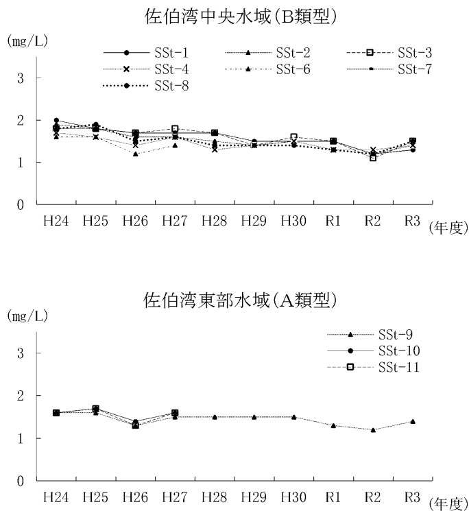
図 g 佐伯湾 COD 年間平均値の経年変化
