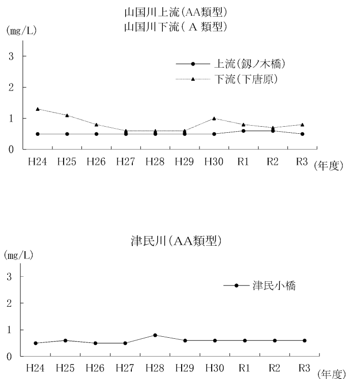
図 a 山国川水系 BOD 年間平均値の経年変化
