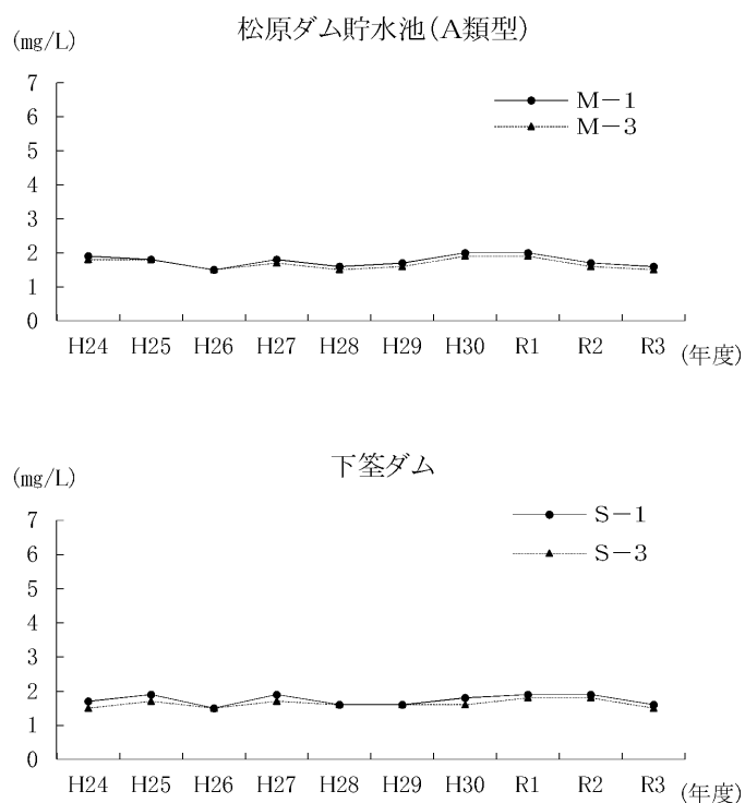
図 各湖沼 COD 年間平均値の経年変化
