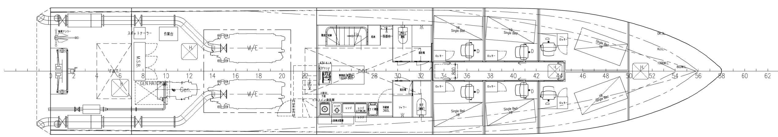
舵機室 機関室 食堂 船員室 船首倉庫
