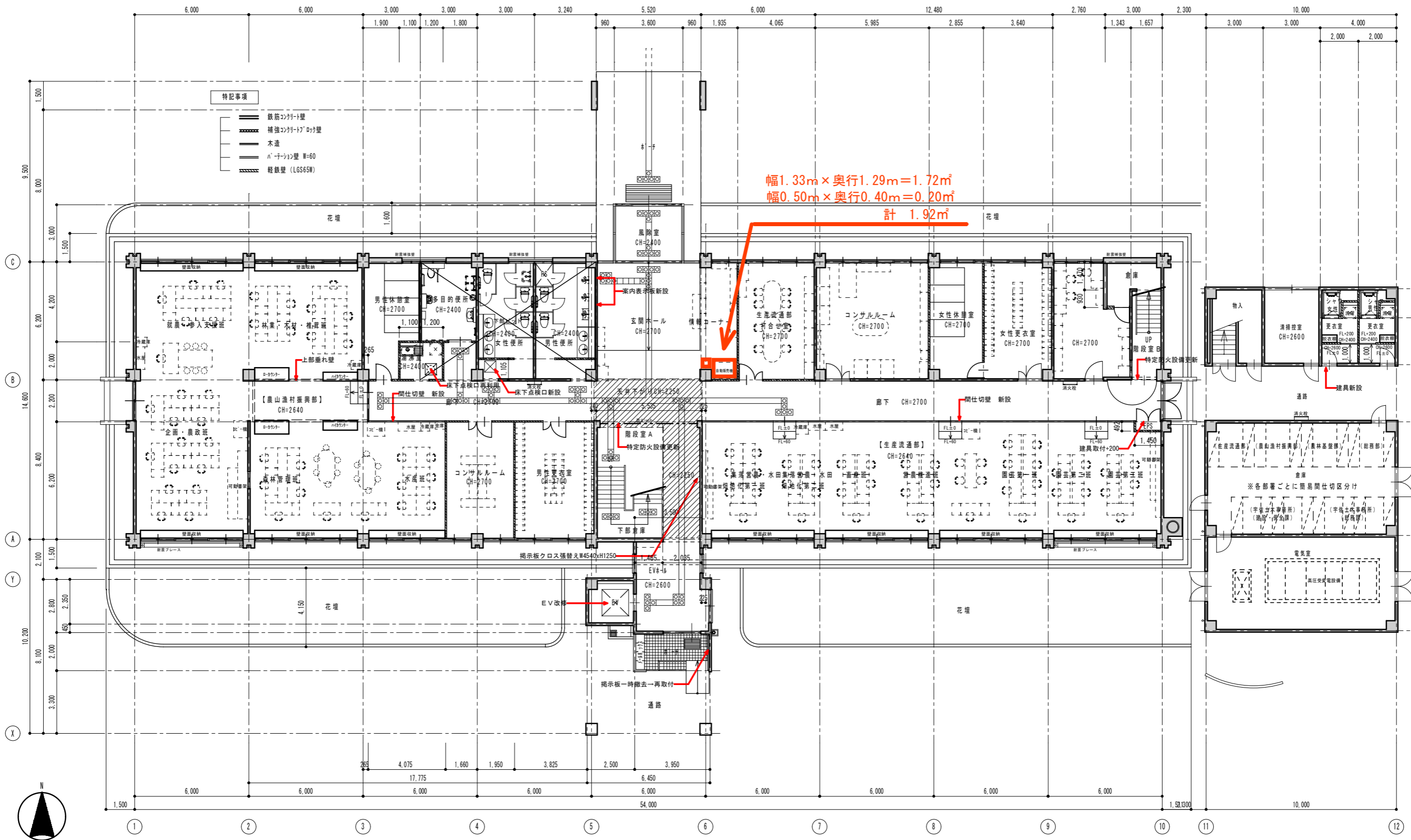
改修1階平面図 S=1/100
