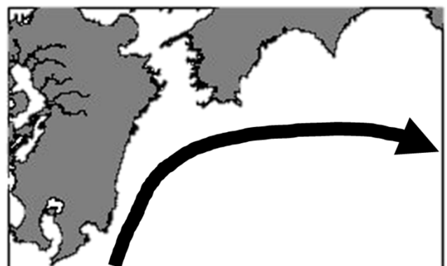
黒潮流路図
