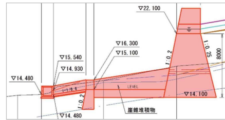
縦断面図
