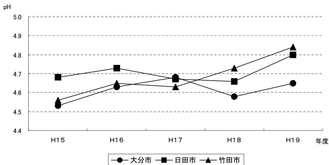
図6-2 雨水のpHの年平均値の経年変化
