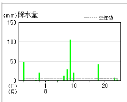
地上気象 気象経過図：2023年07月25日-2023年08月24日
