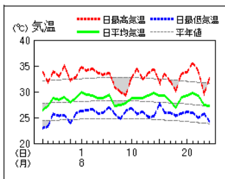
地上気象 気象経過図：2023年07月25日-2023年08月24日
