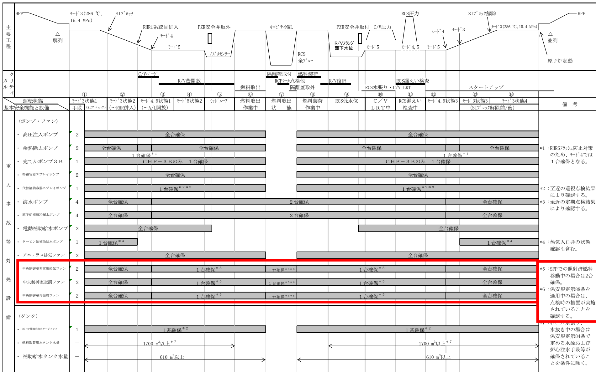
原子炉停止時の安全機器等の待機状態図（重大事故等対処設備に係わる安全措施）
