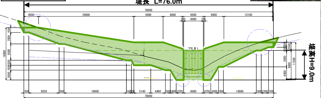
施工計画図
