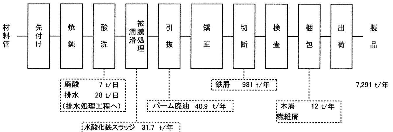
図1 冷間引抜き鋼管製造フローシート
