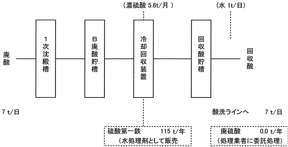
図2 廃酸回収フローシート
