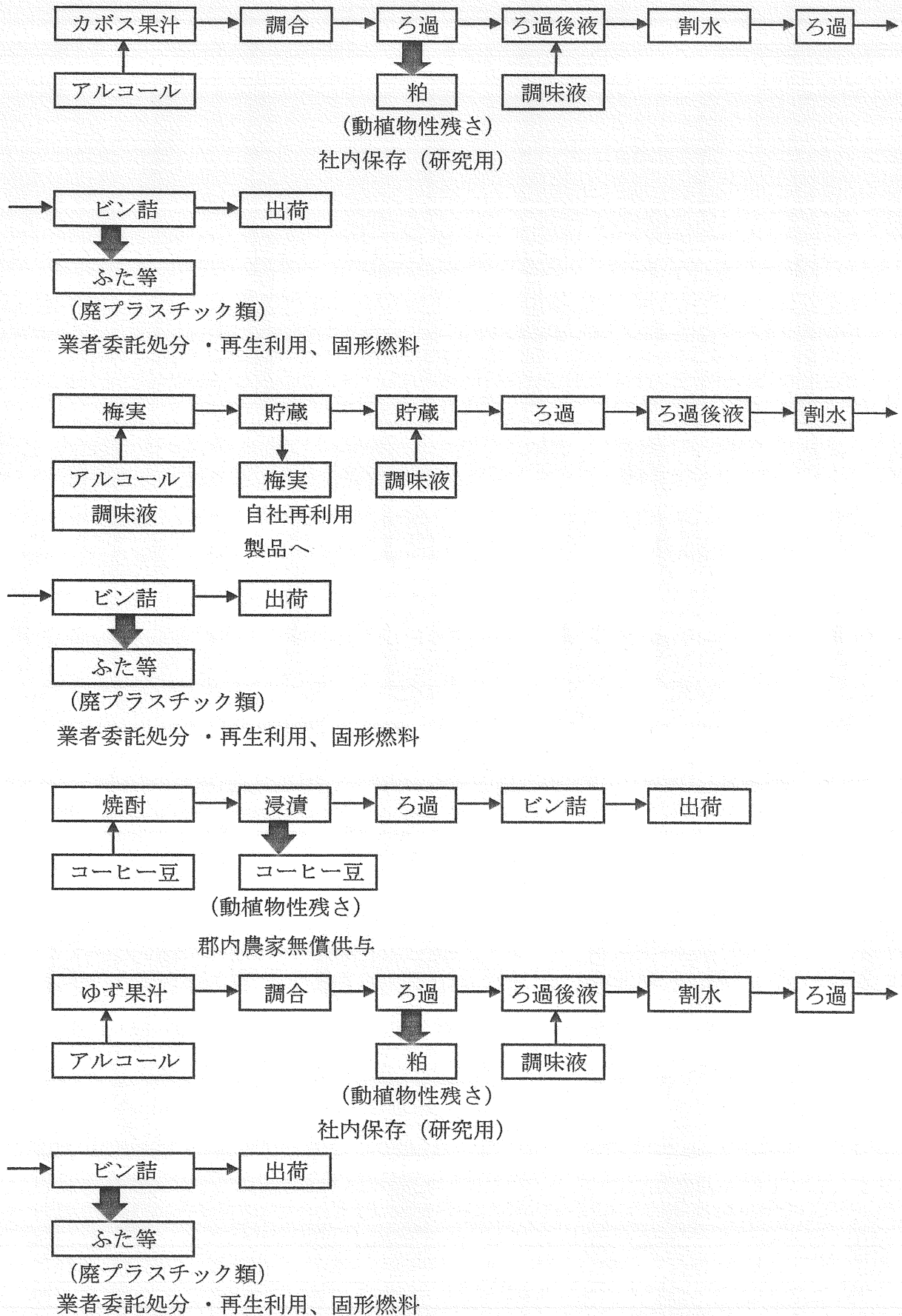
図3 リキュール製造フローシート
