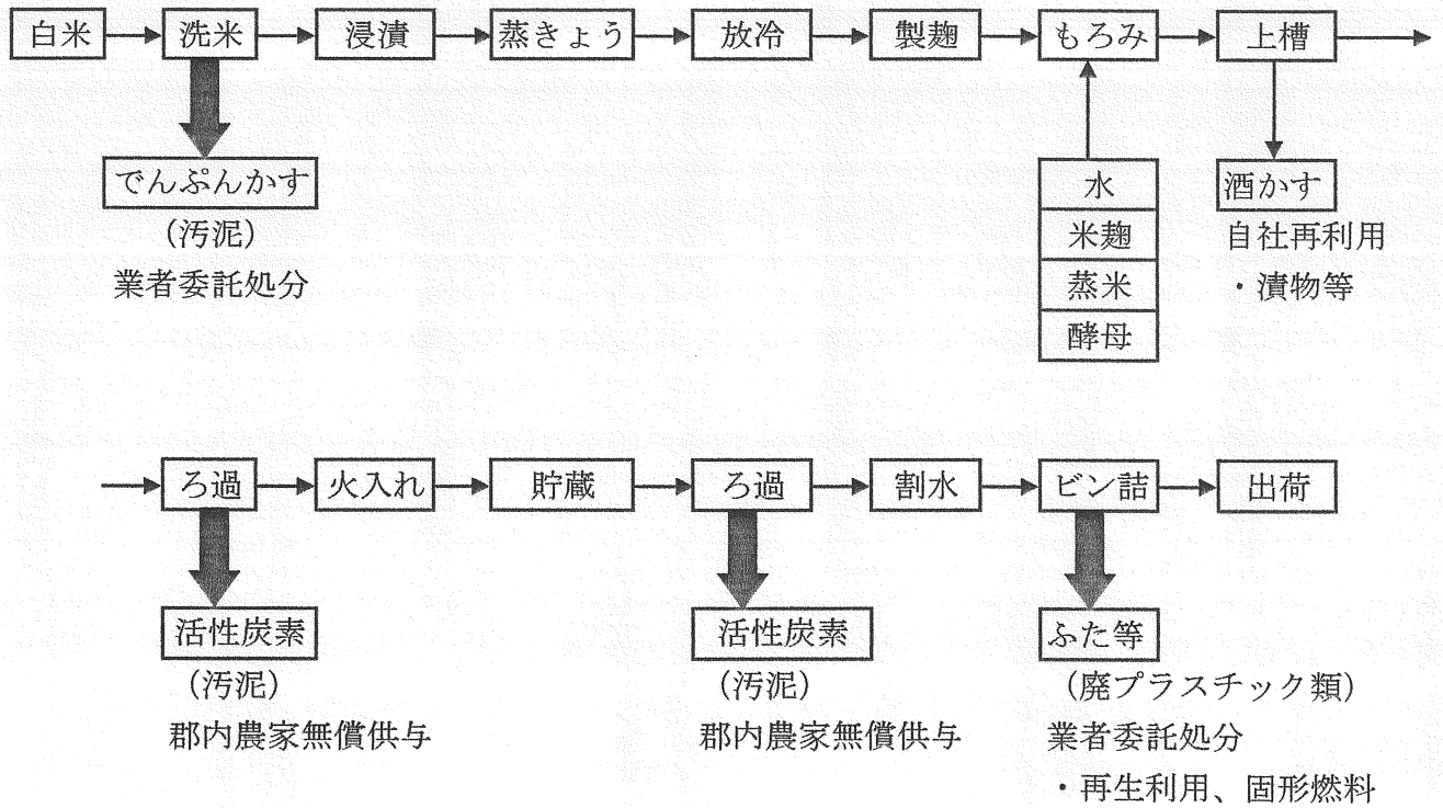
図1 清酒製造フローシート
