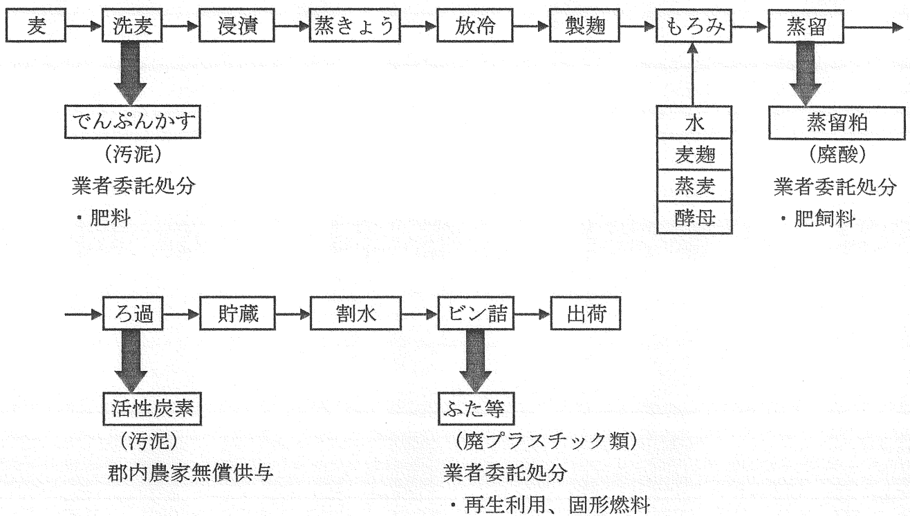
図2 焼酎製造フローシート
